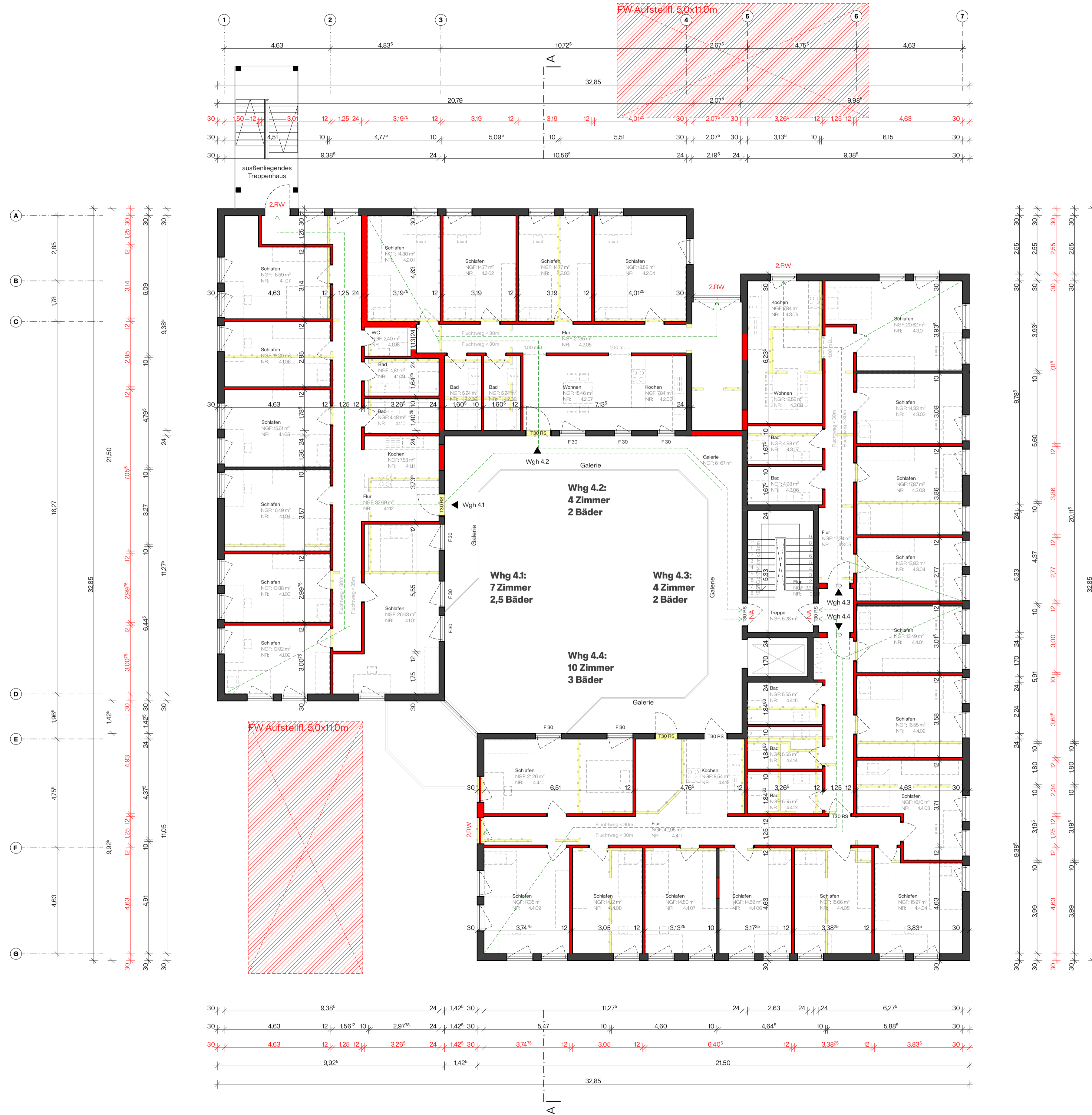
Grundriss 4 Obergeschoss | M 1:100
