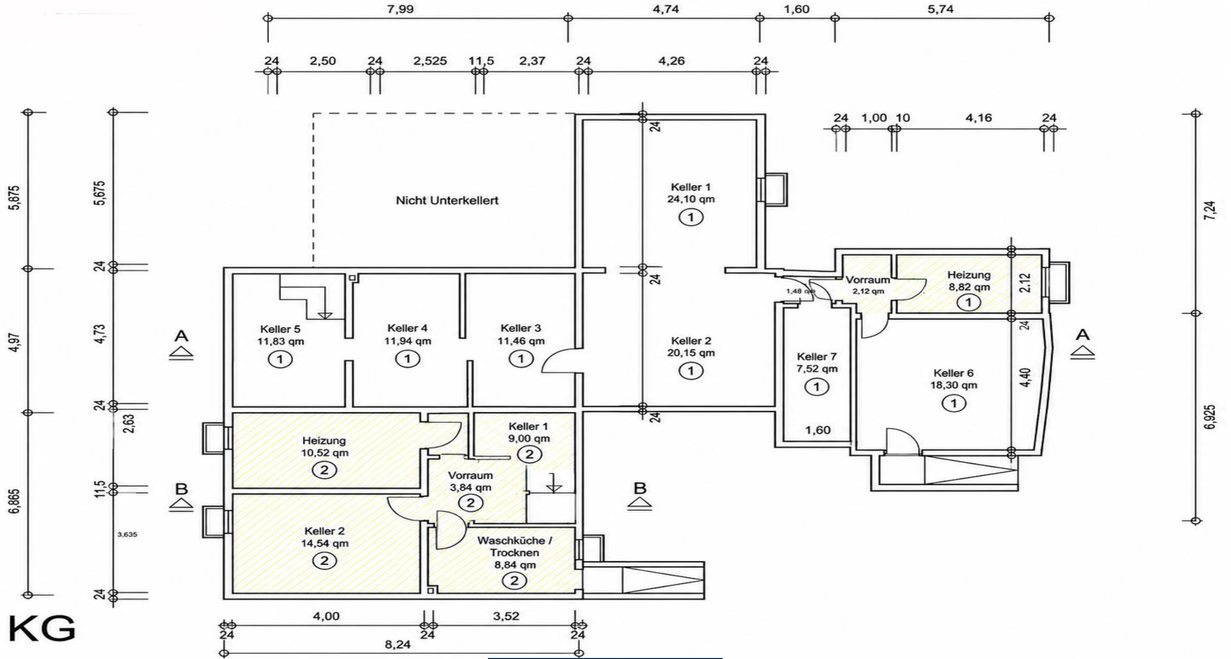
Grundriss KG
