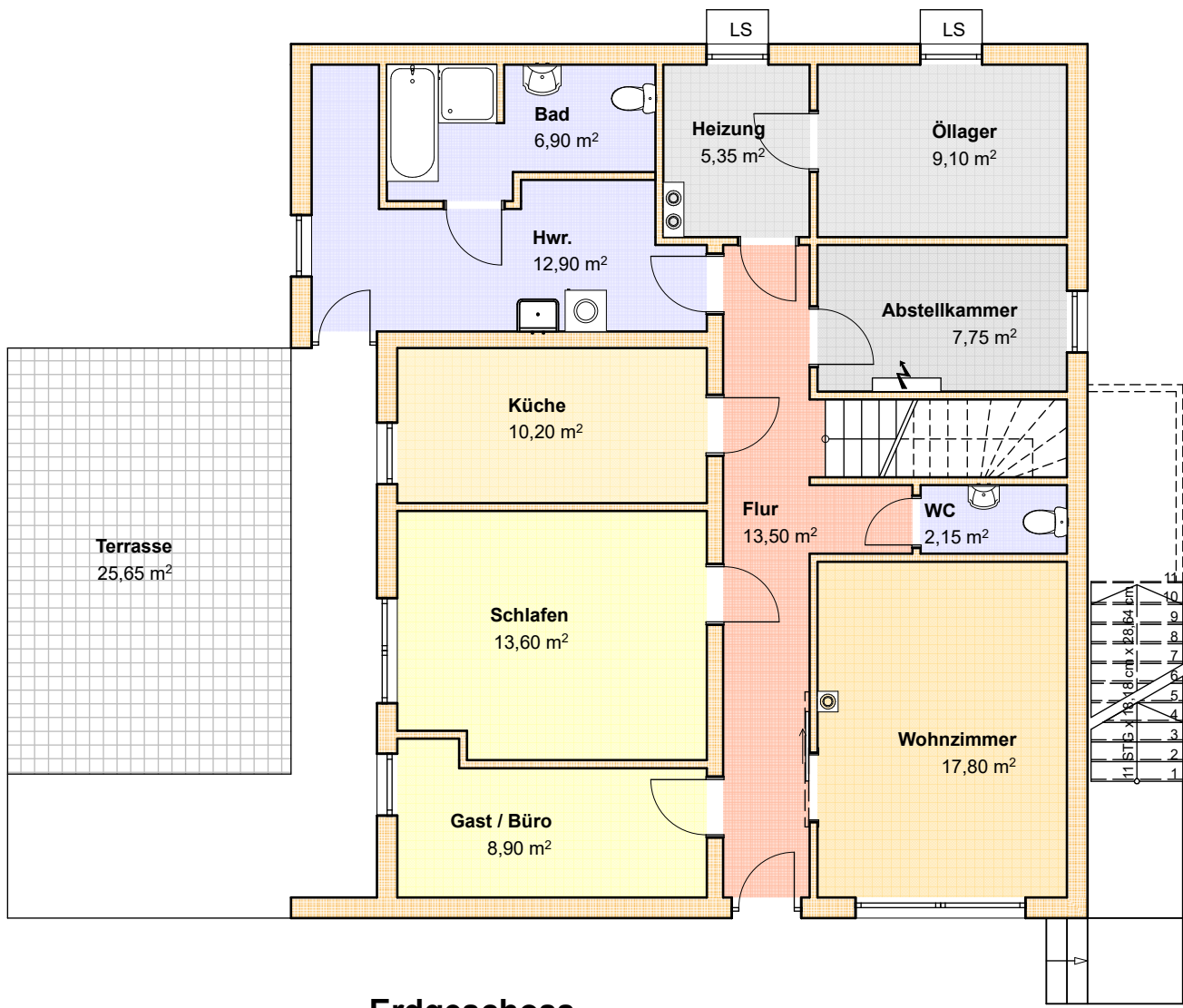
Erdgeschoss
