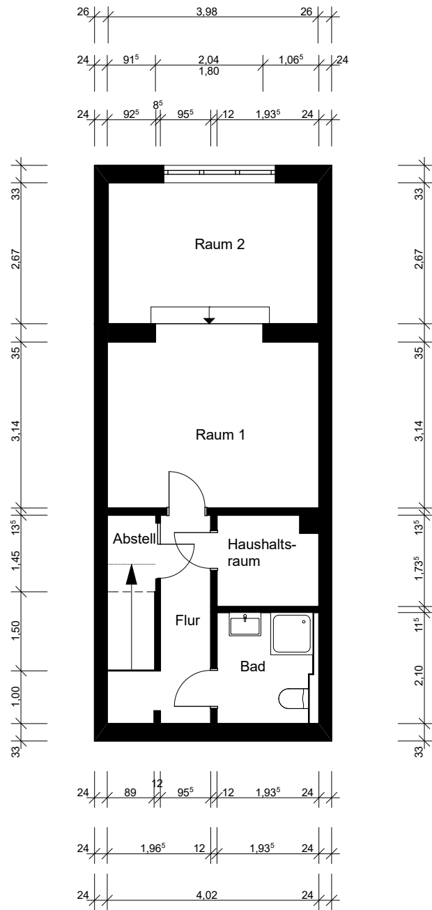
Reihenhaus im Stübekamp Grundriss - Untergeschoss
