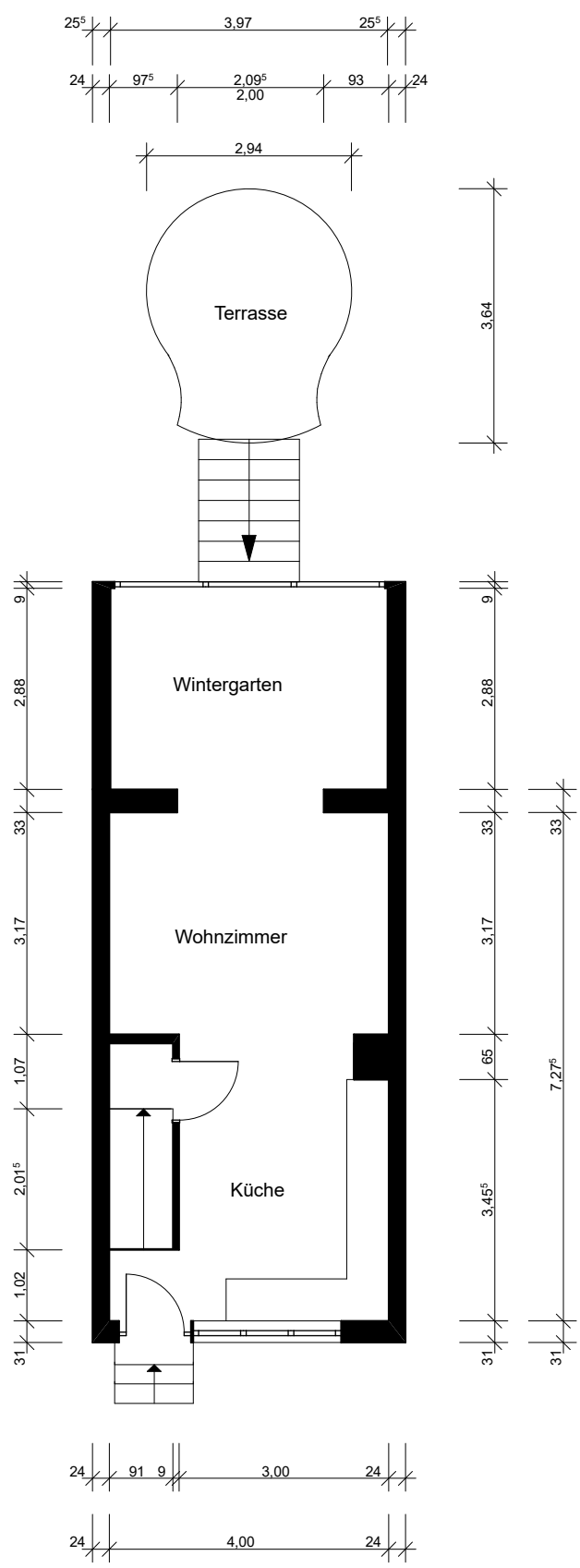
Reihenhaus im Stübekamp Grundriss - Erdgeschoss
