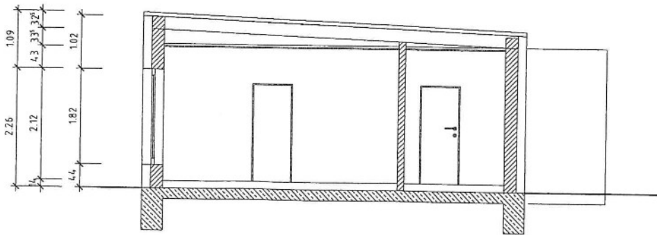
SCHNITT A-A
