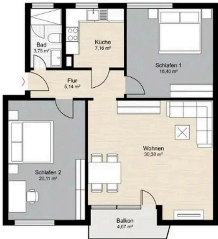
Grundriss
