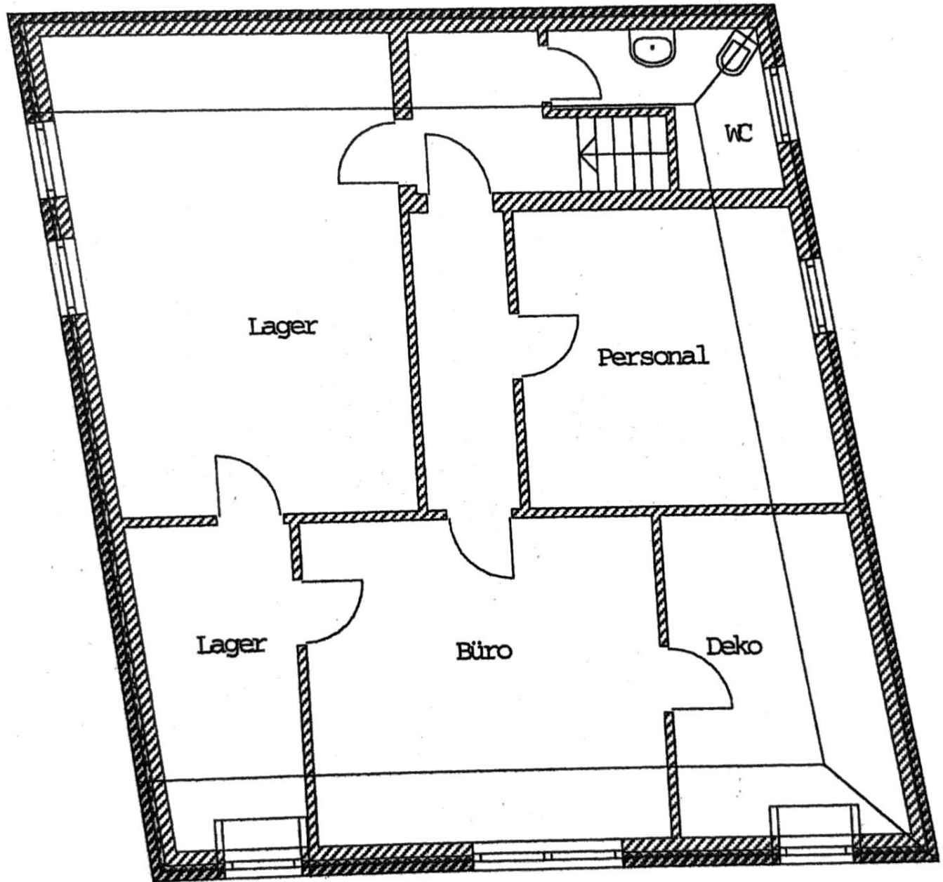
Dachgeschoß M. 1:100
