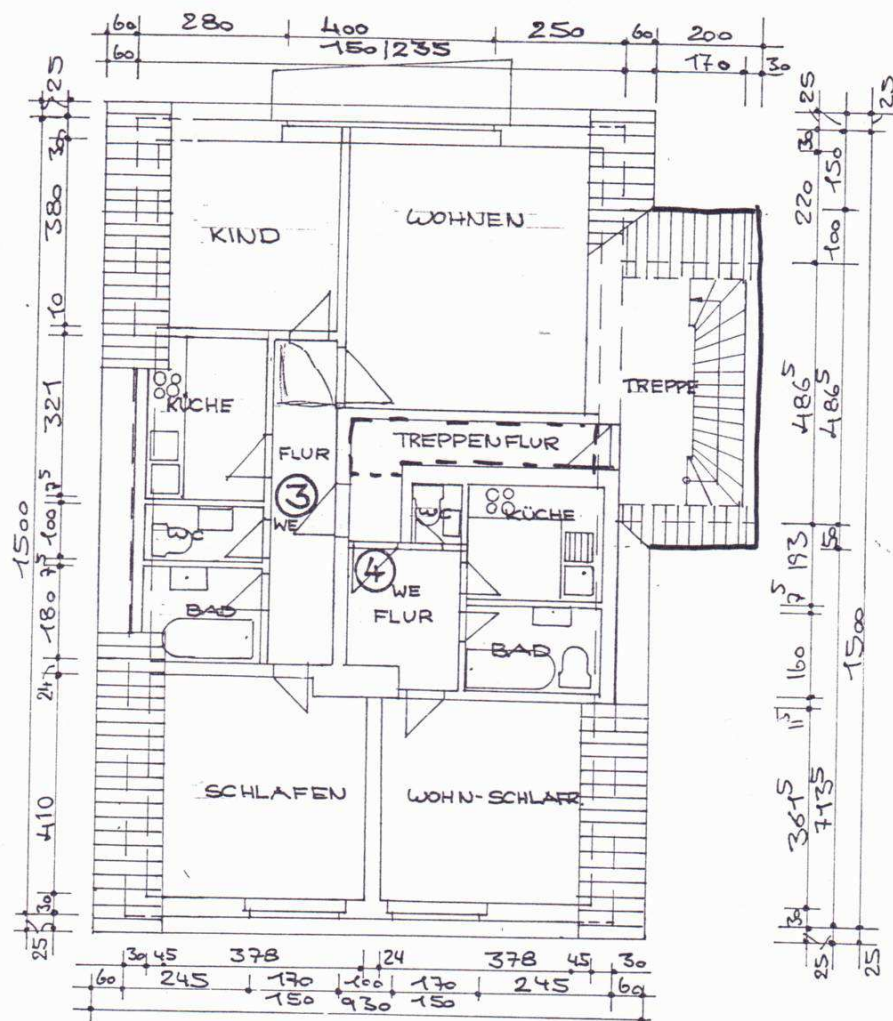
DACHGESCHOSS M 1:100
