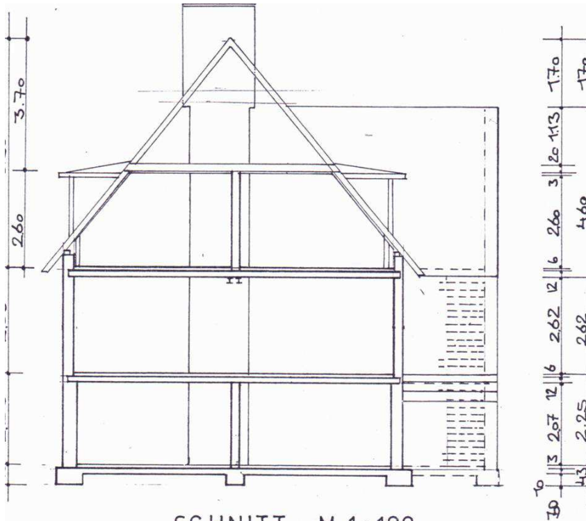
SCHNITT M 1:100
