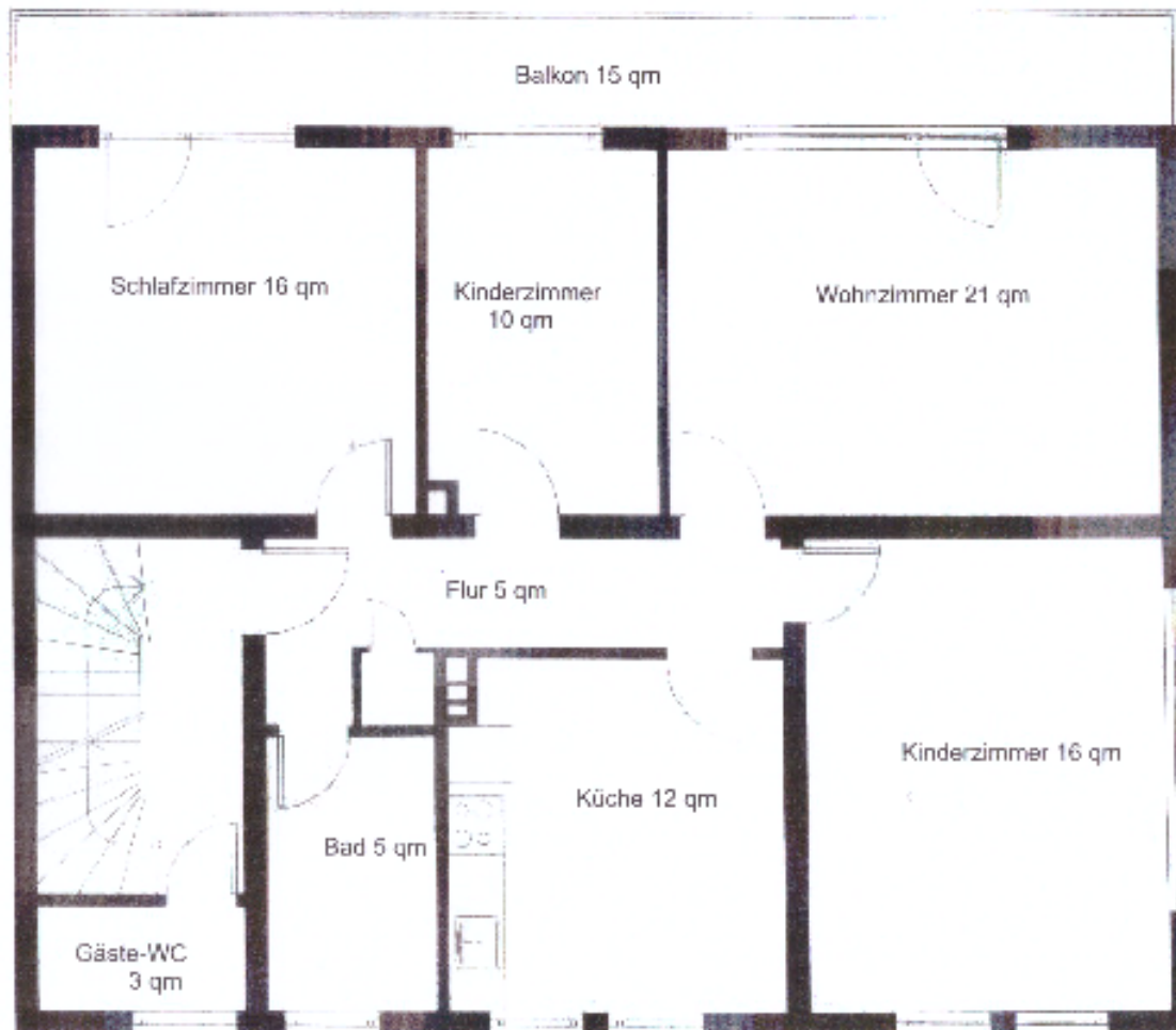
Obergeschoss
