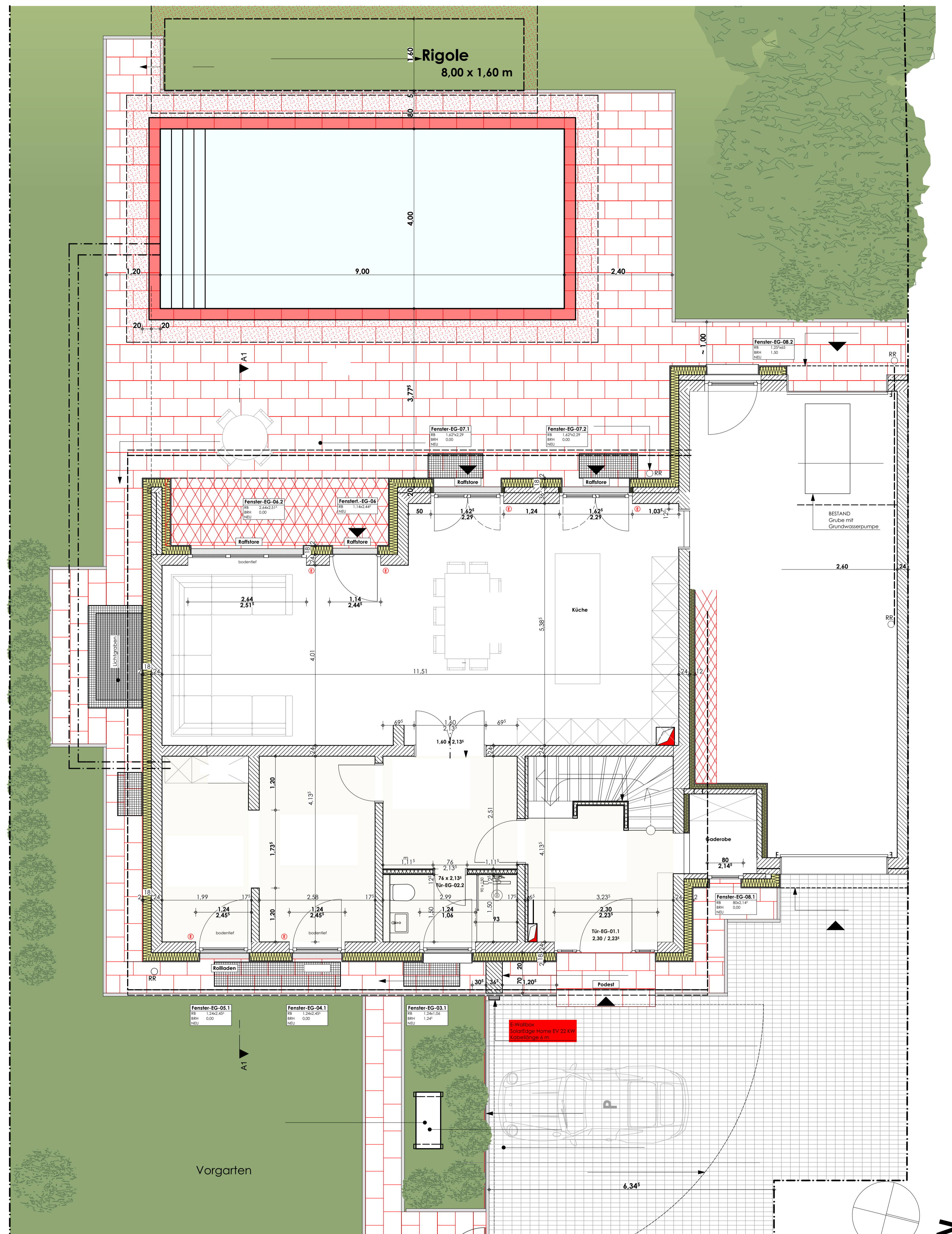
GRUNDRISS EG
