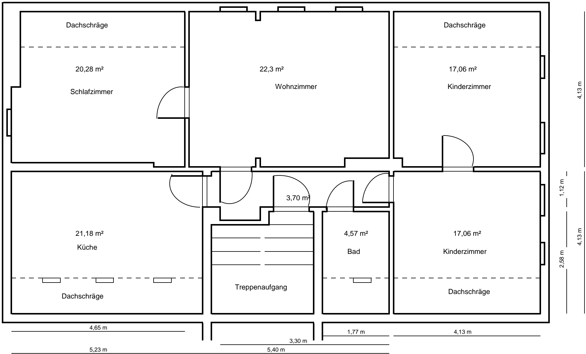
Dachgeschoss Wohnung ca. 100 m 2
