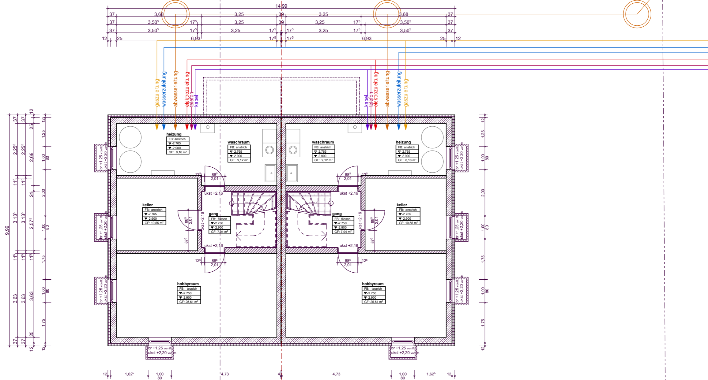
kellergeschoss doppelhaus 1 kellergeschoss doppelhaus 1
