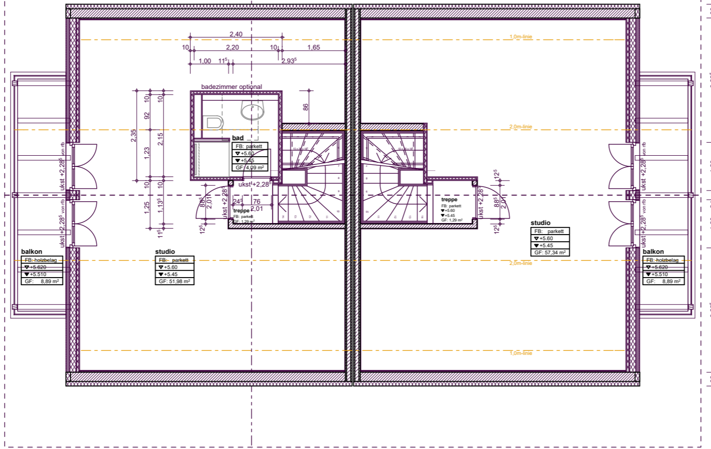
dachgeschoss doppelhaus 1
