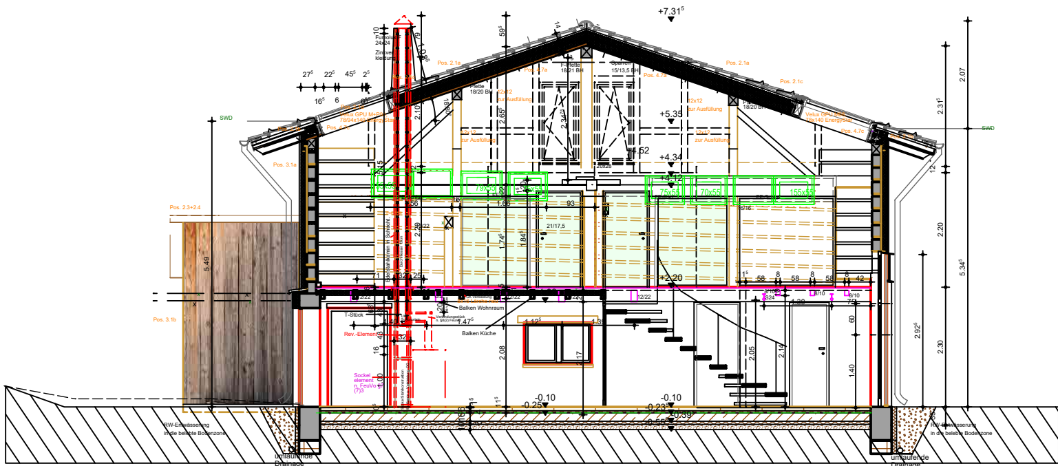
SCHNITT b-b SCHEUNE/STALL
