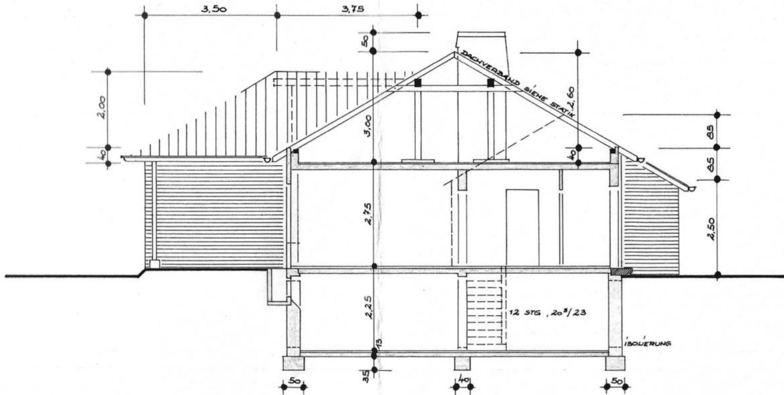
QUERSCHNITT
