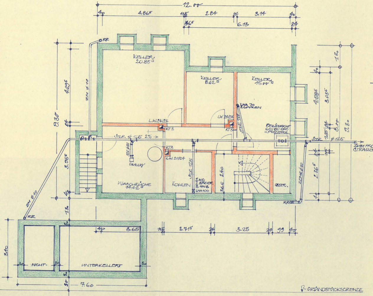
KELLERGRUNDRISS:
