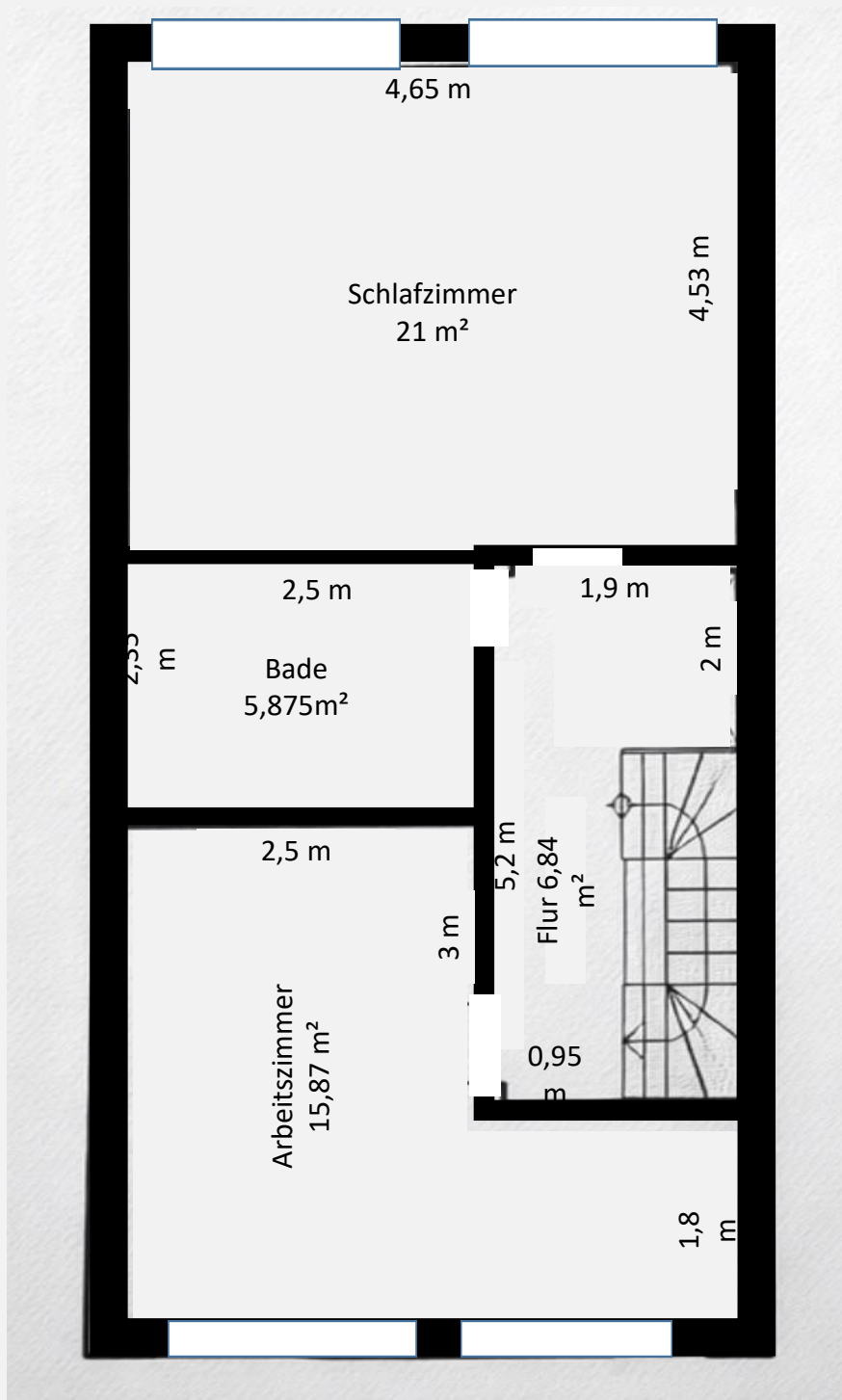
Obergeschoss 49,58 m 2
