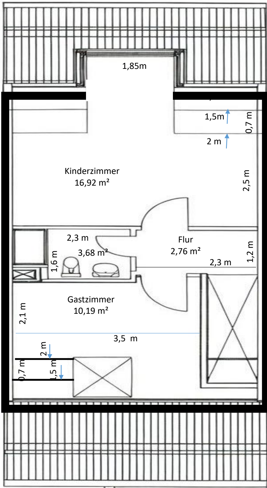
Dachgeschoss 33,55 m 2
