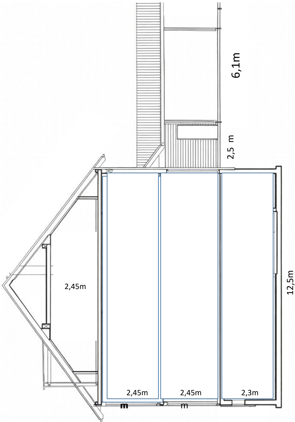
Schnitt
