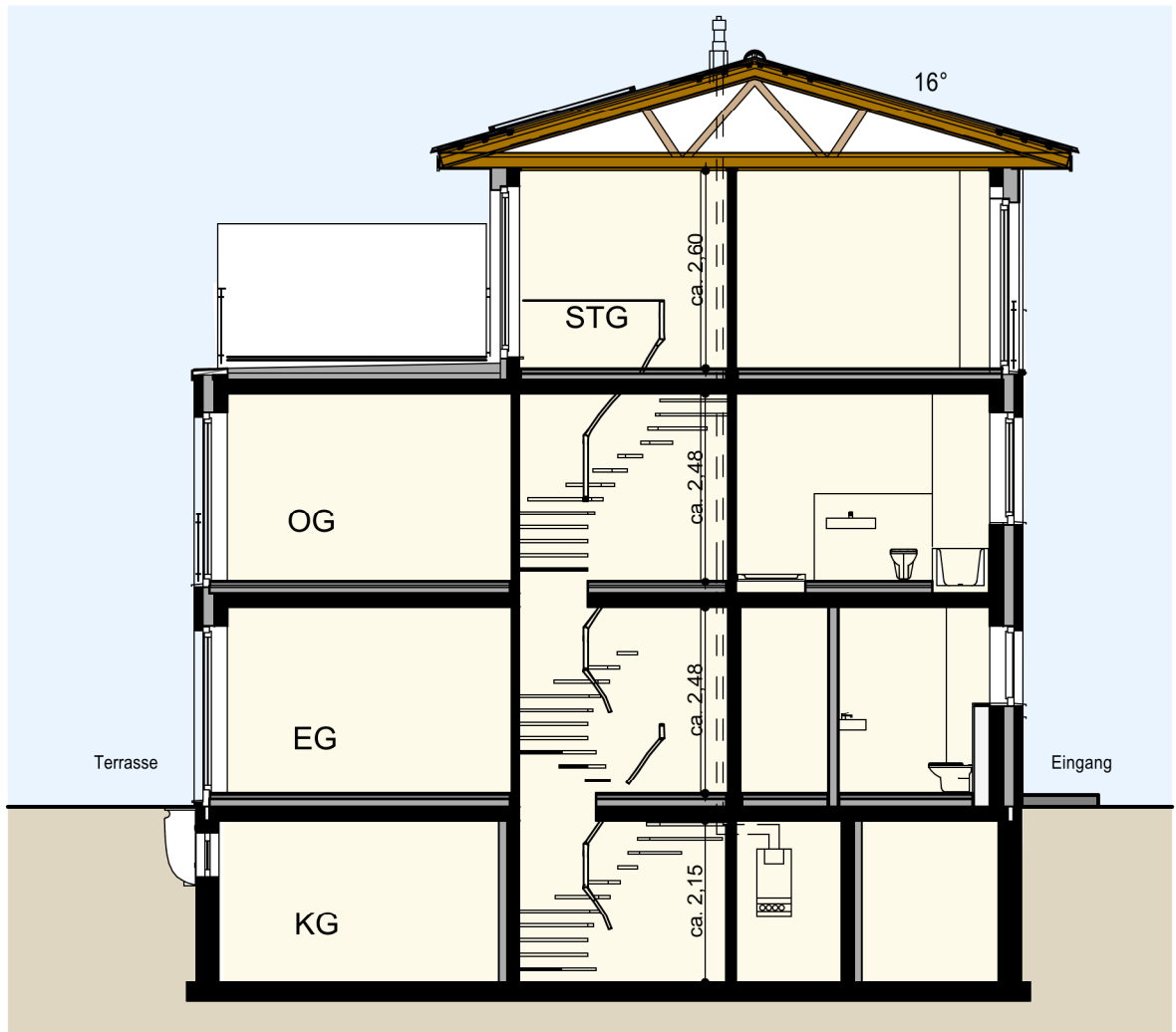
Schnitt
