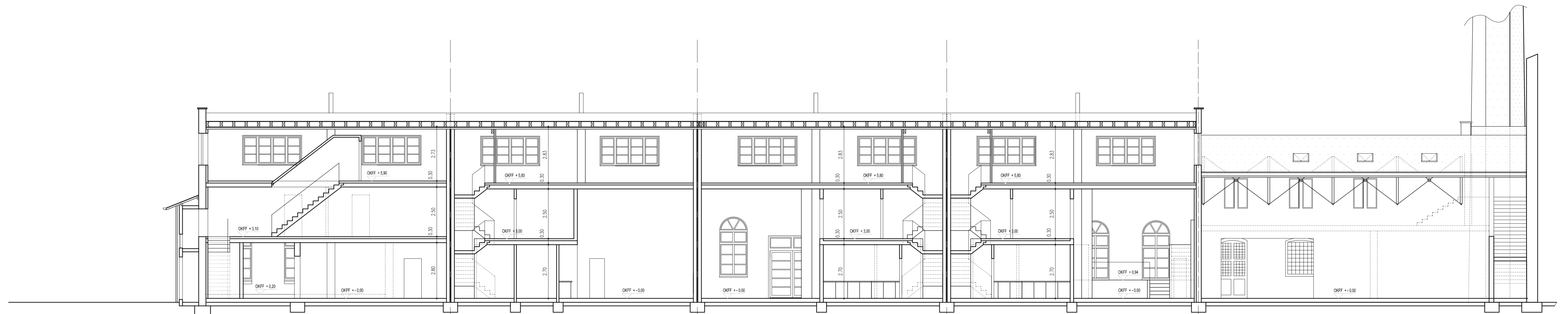
Längsschnitt L
