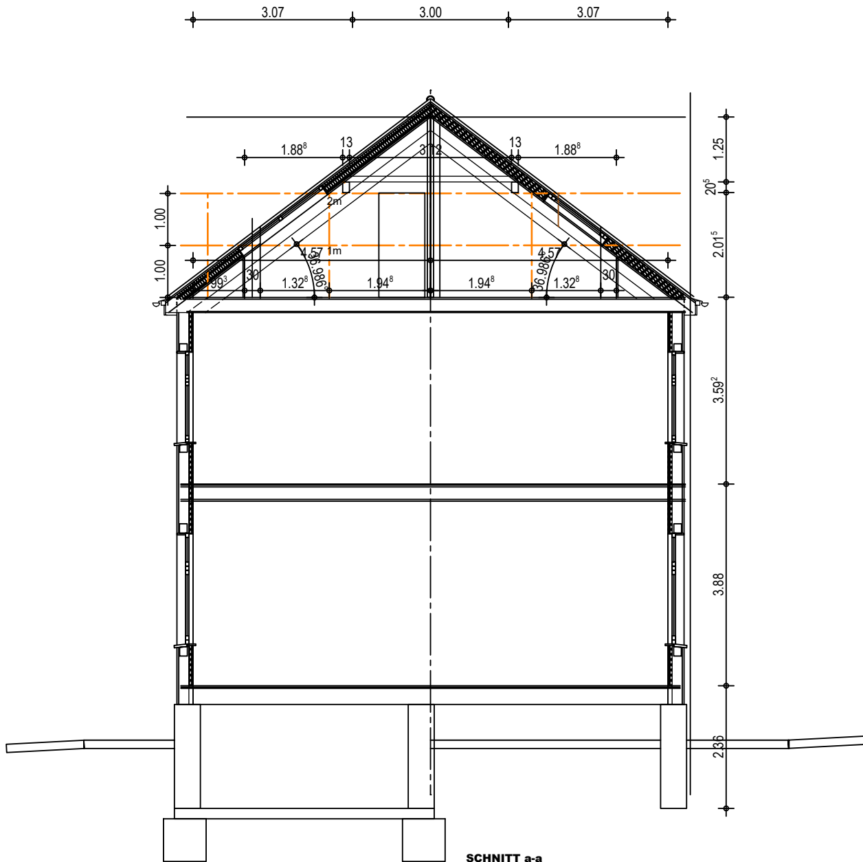
SCHNITT a-a
