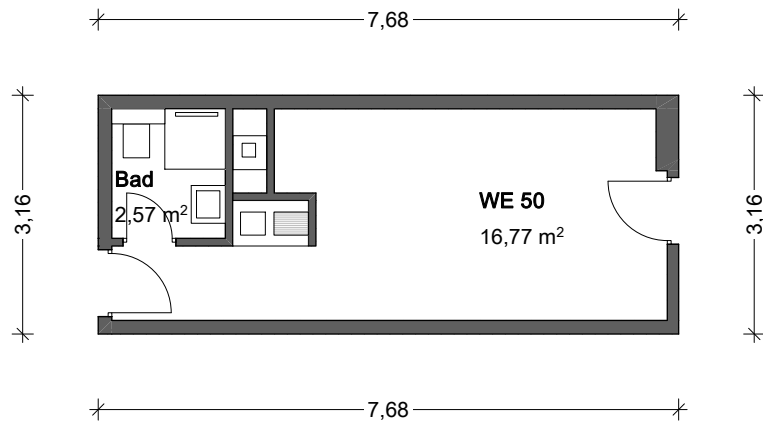
Mit basic Masskette
