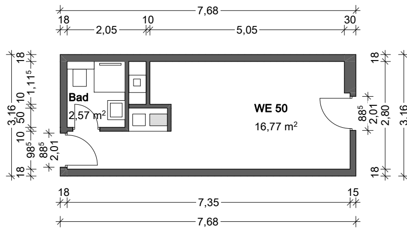
Mit detaillierte Masskette
