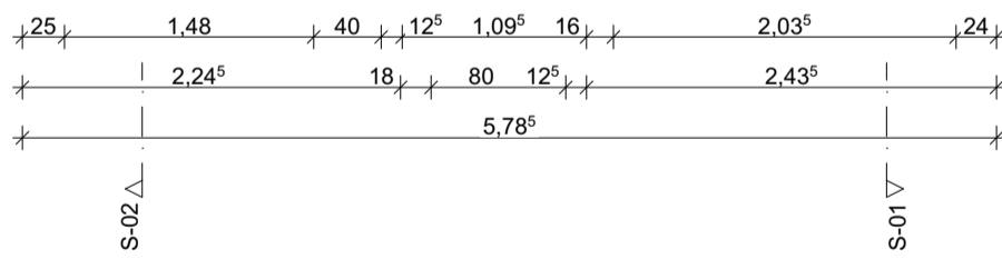
Grundriss
