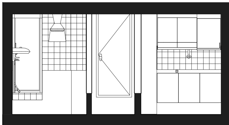
Schnitt -04
