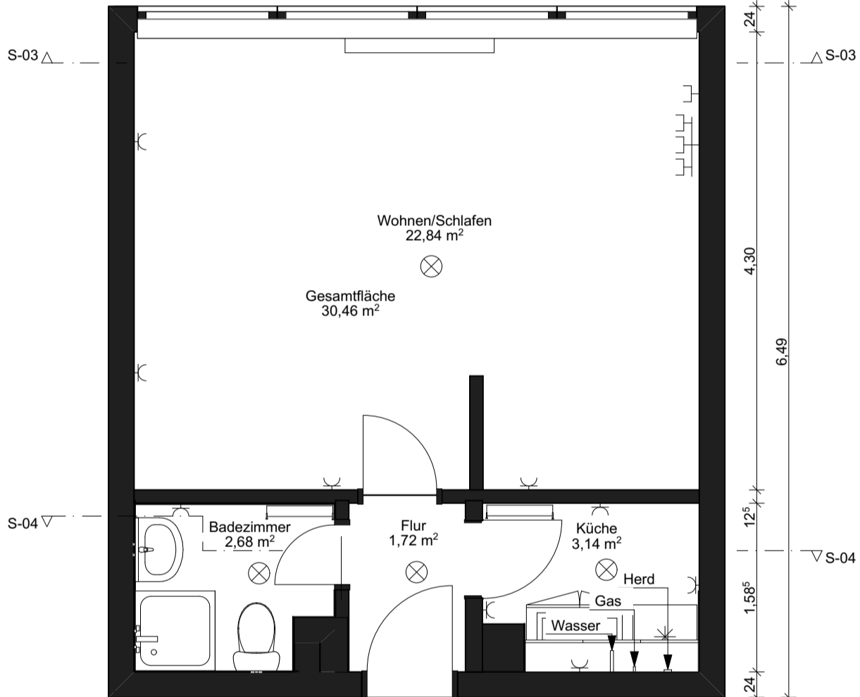
Grundriss
