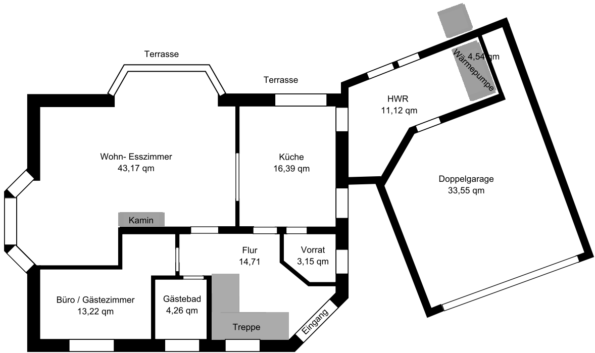
Nicht maßstabsgetreuer Grundriss Erdgeschoss
