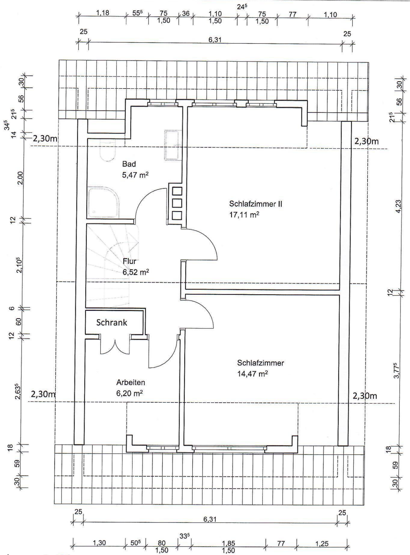
Dachgeschoss 1:50
