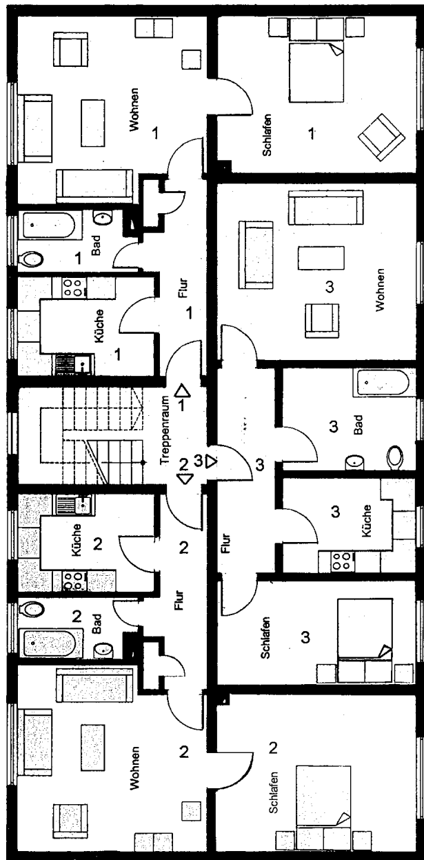
Erdgeschoss M 1: 100
