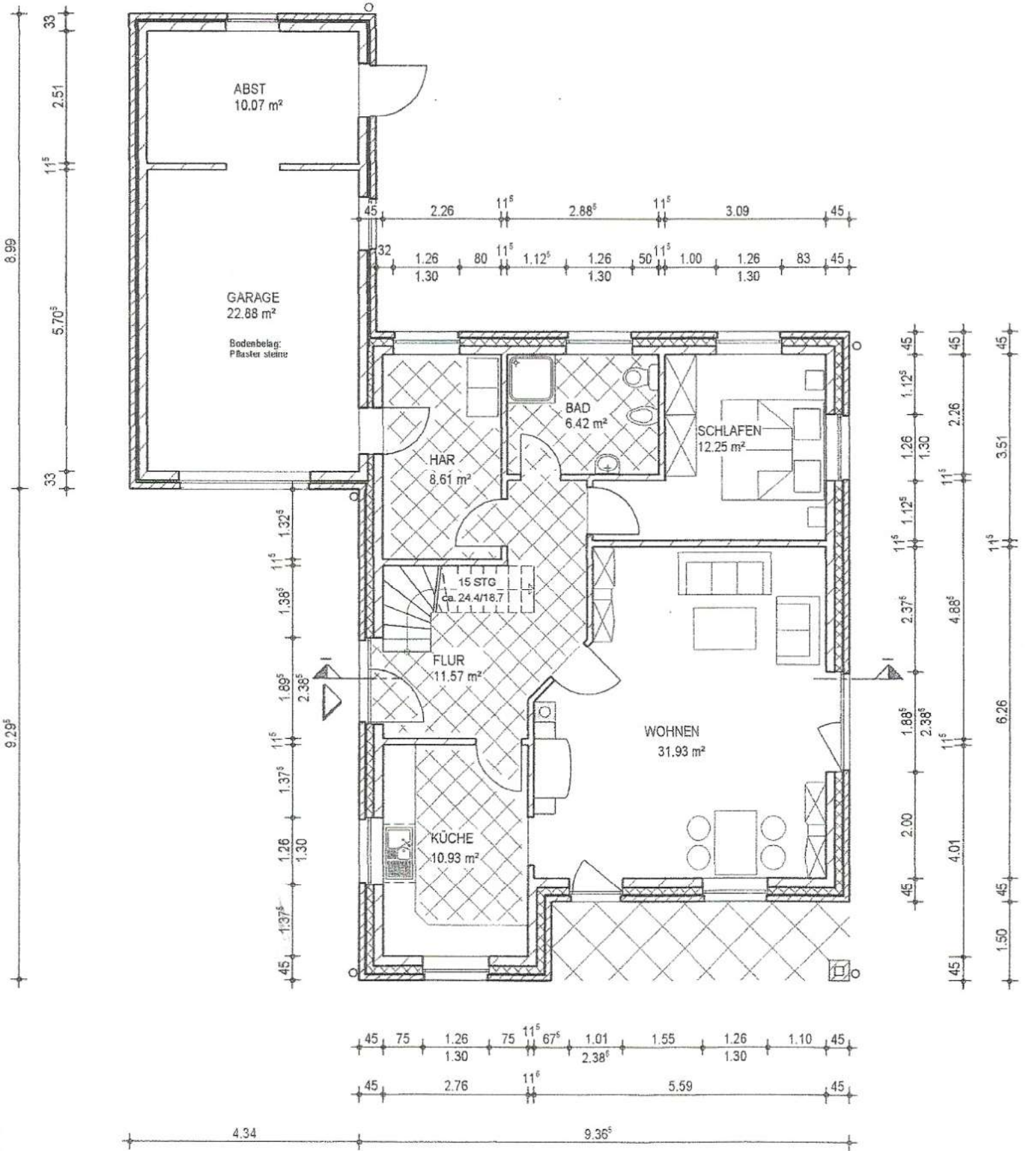
ERDGESCHOSS
