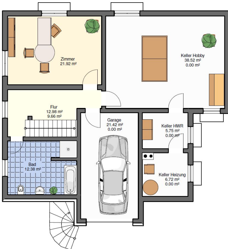
Grundriss Kellergeschoss
