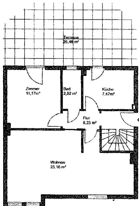
Grundriss Erdgeschoss
