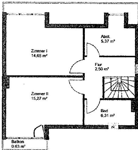
Grundriss Dachgeschoss
