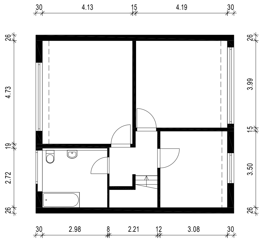
Obergeschoss
