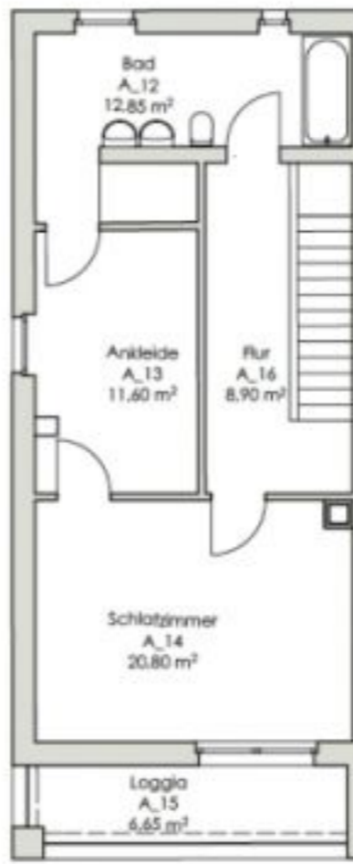
2.Obergeschoss 1:100
