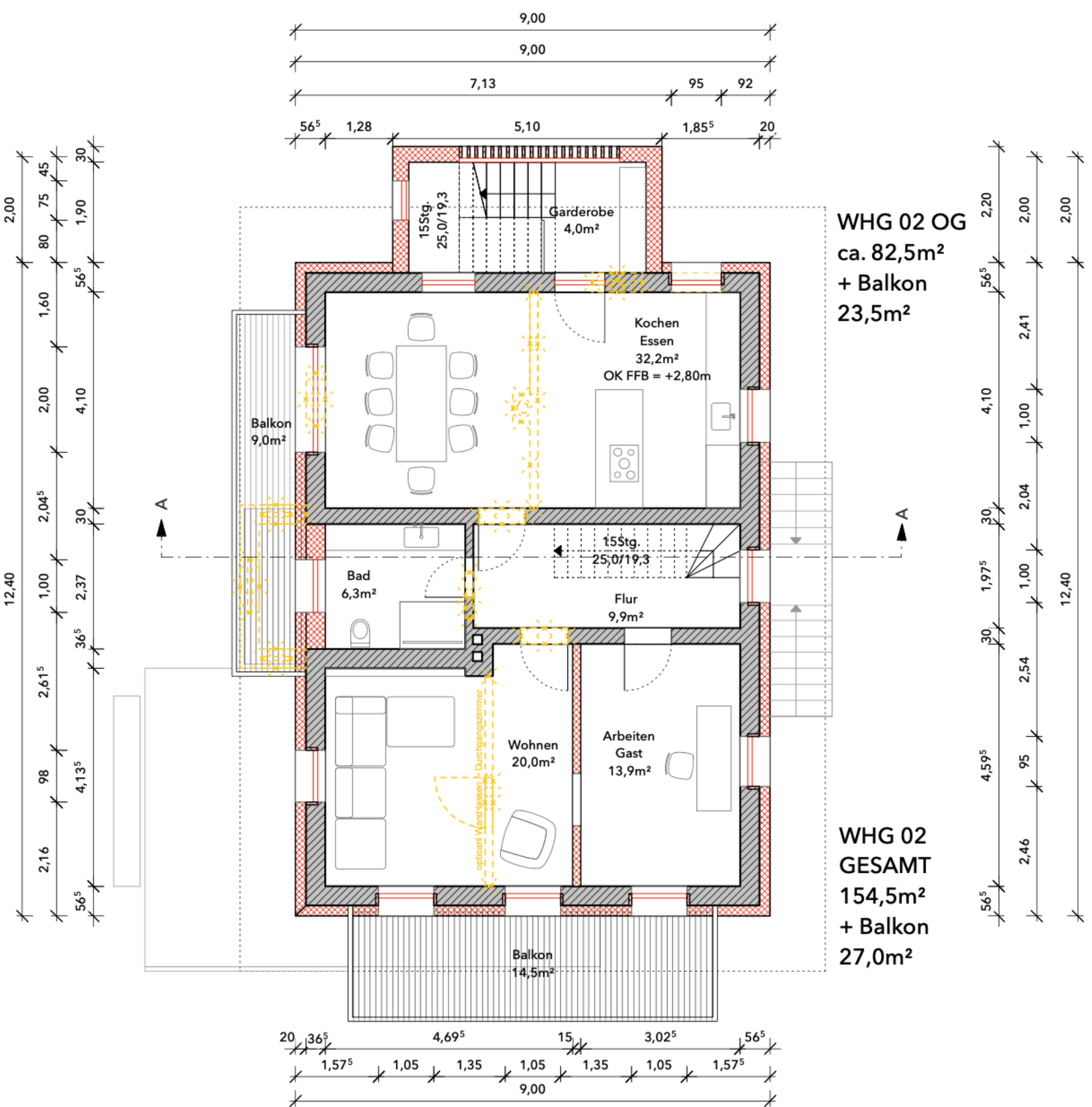
GRUNDRISS OG M 1/100
