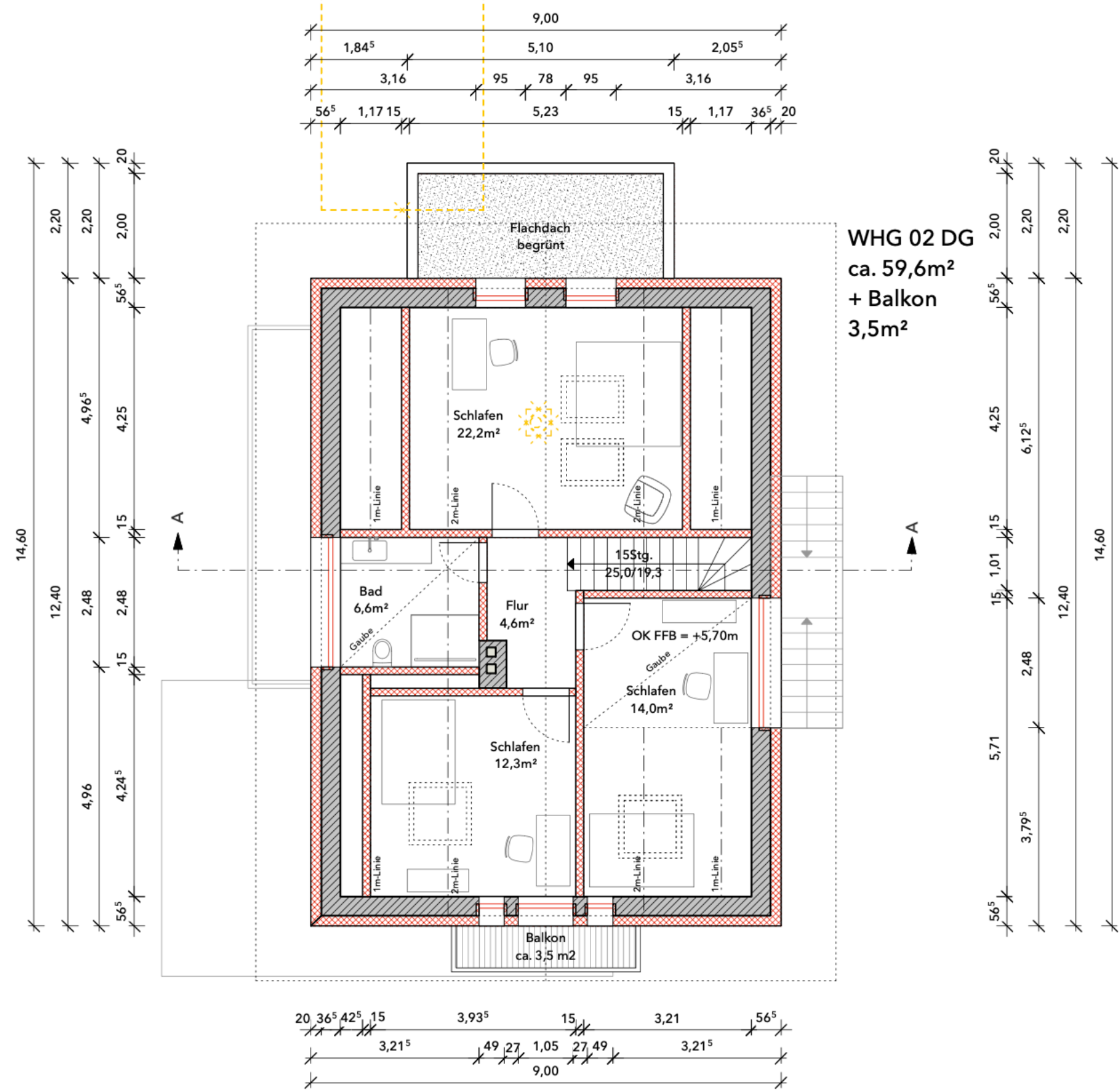
GRUNDRISS DG M 1/100
