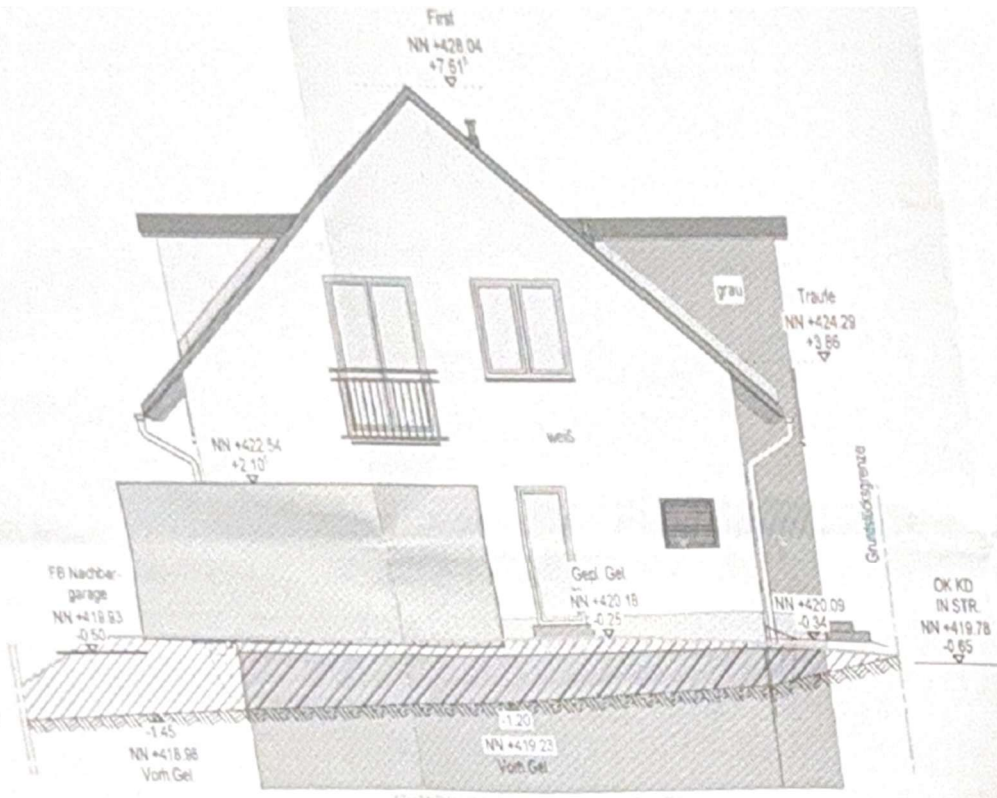
ANSICHT OST (Gelände an Grenze)
