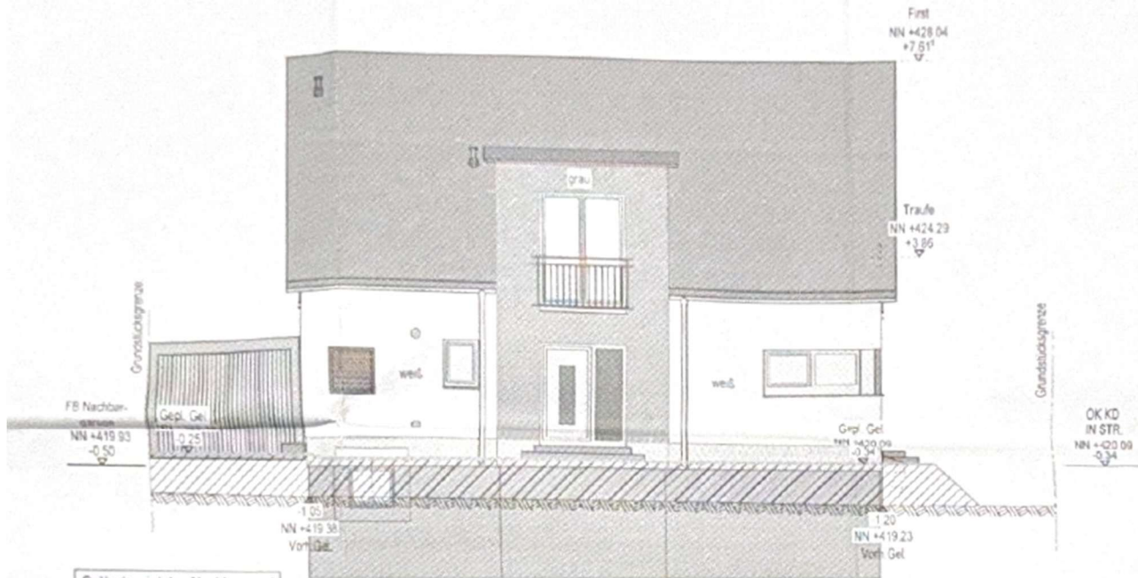
ANSICHT NORD
