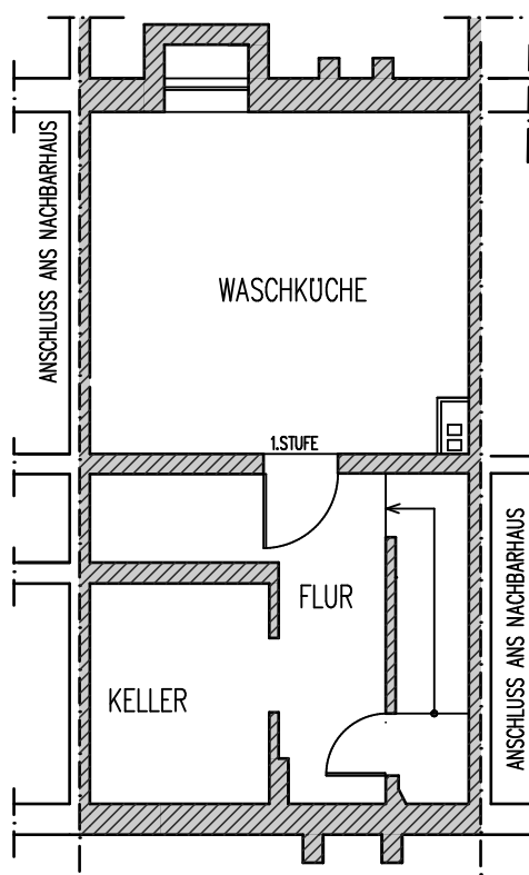
KELLERGESCHOSS-GRUNDRISS
