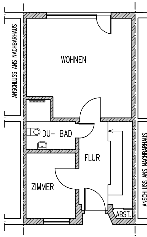
ERDGESCHOSS-GRUNDRISS
