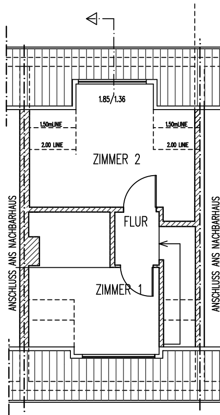
DACHGESCHOSS-GRUNDRISS
