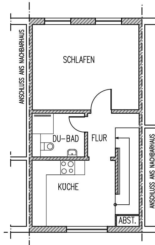
OBERGESCHOSS-GRUNDRISS
