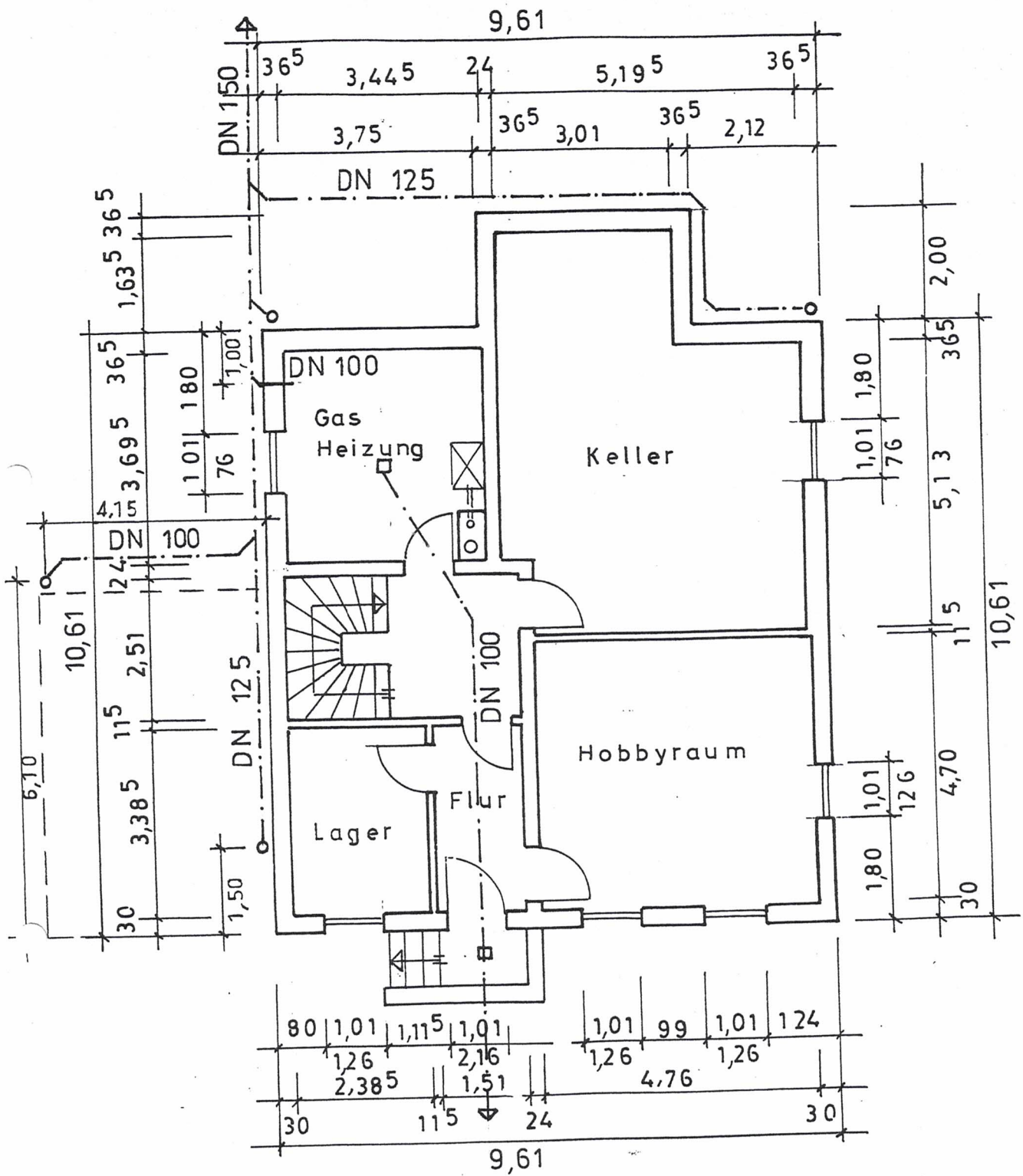
Kellergeschoß
