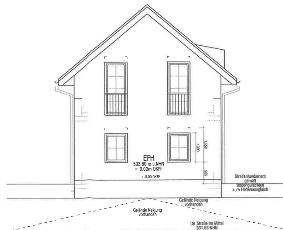
Ansicht 2 Nord
