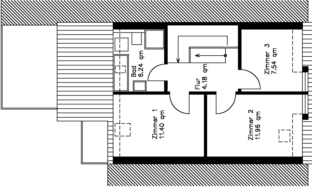
Dachgeschoss, 41.32 qm Wfl.
