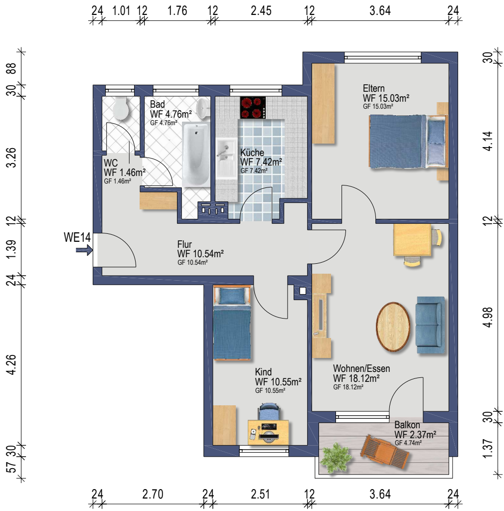
1.Obergeschoss
