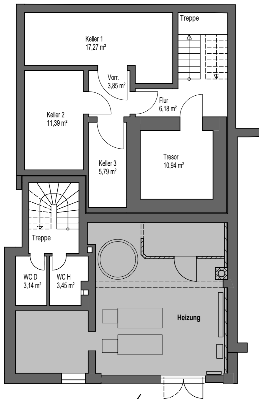
Keller
