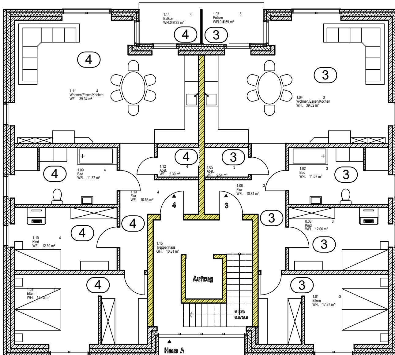
Obergeschoss M 1:100 Haus A
