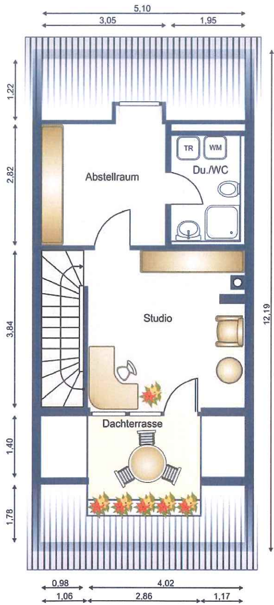
Grundriss Dachgeschoss
