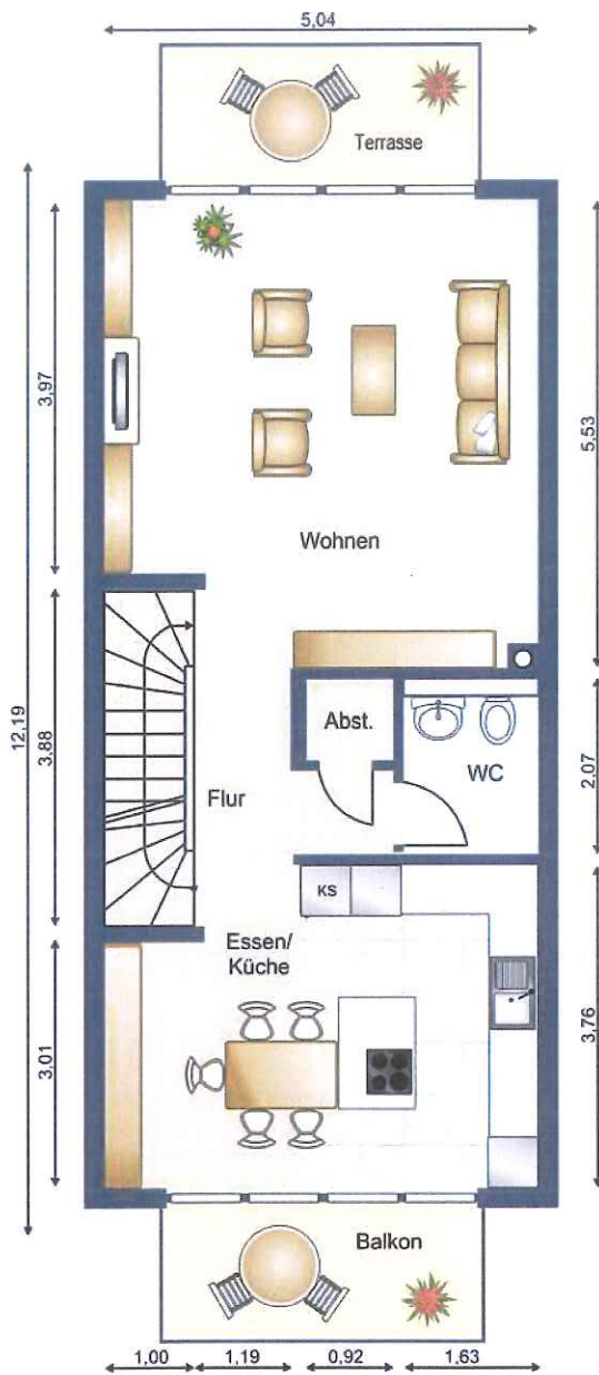
Grundriss Erdgeschoss
