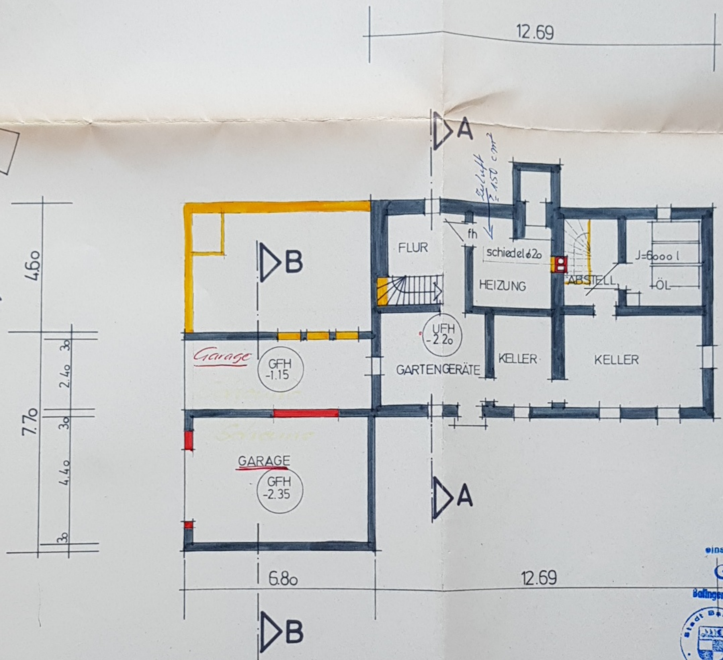
UNTERGESCHOSS M. 1/100
