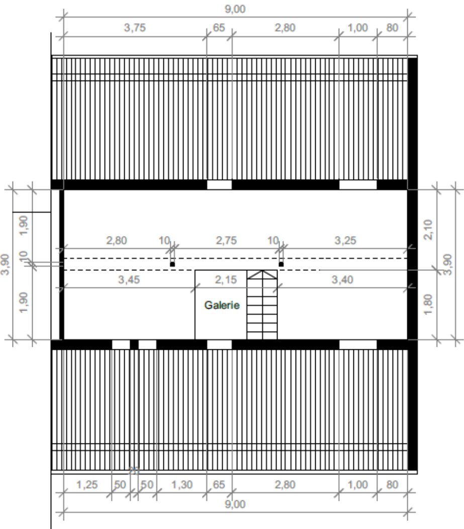
4 Obergeschoss
