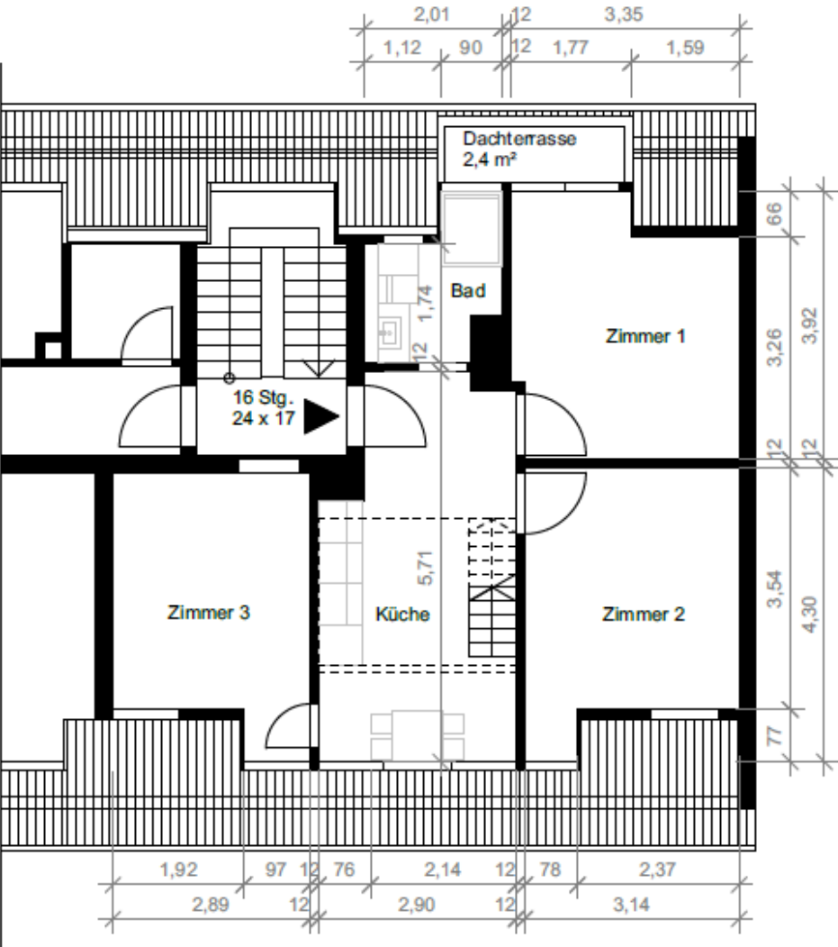
3 Obergeschoss
