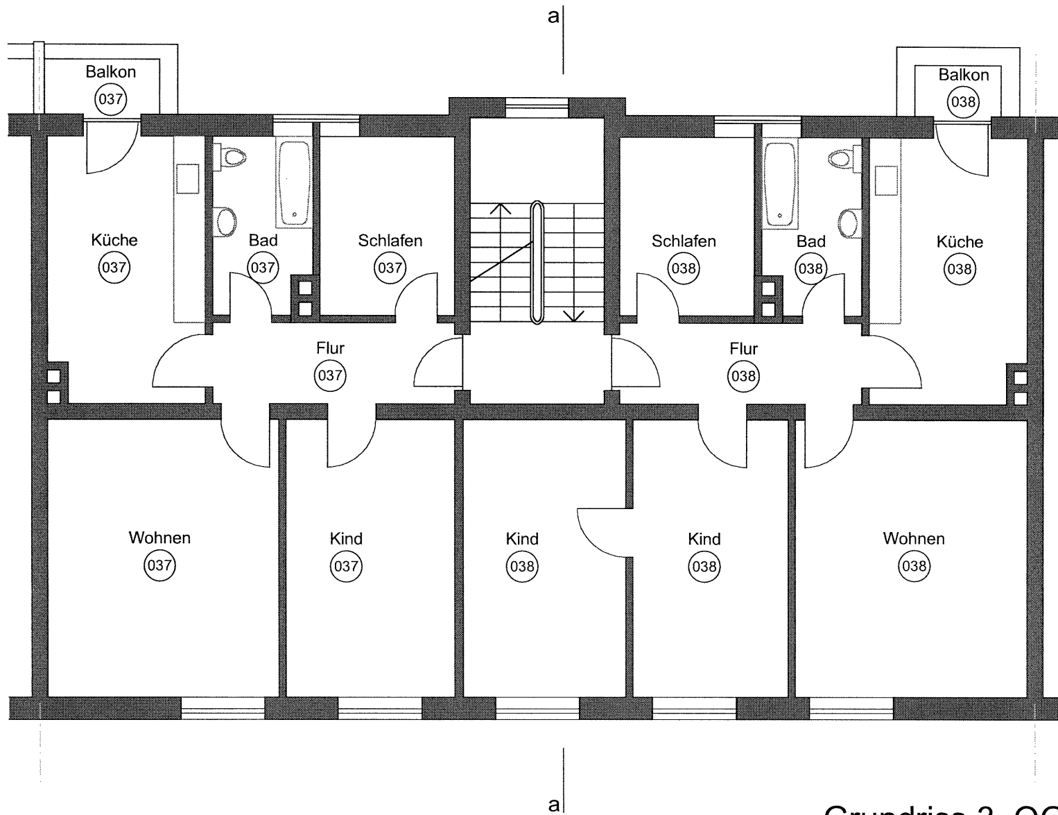
Grundriss 3. OG
