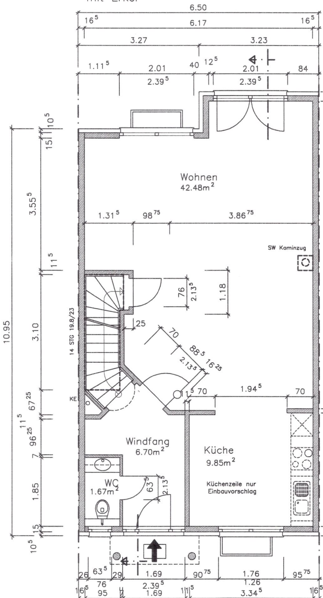
ERDGESCHOSS mit Erker
