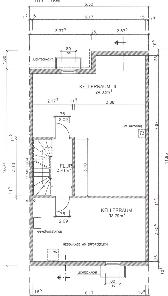
KELLERGECHOSS mit Erker
