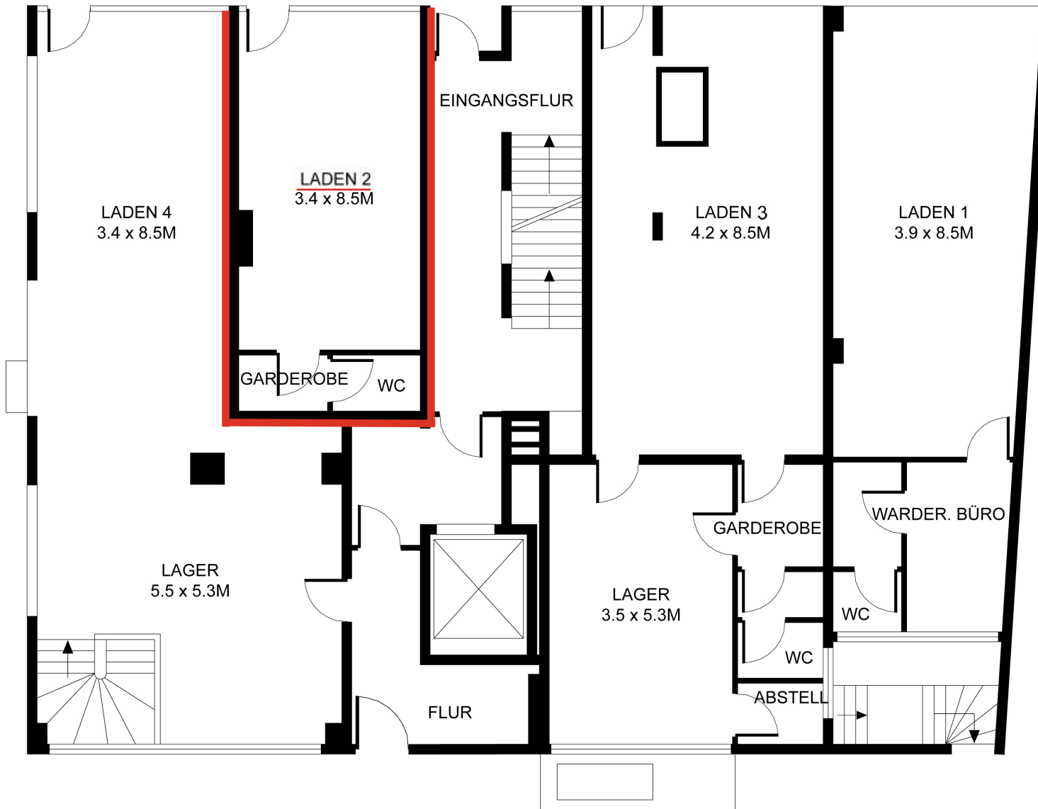
PLANUNG EG
